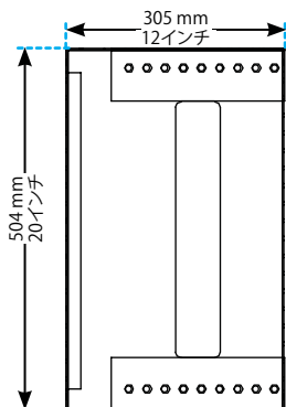
トップビュー 最小深さ
